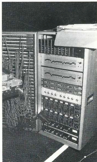
Rack garni dbx, Klark Teknik, filtres BSS etc... à gauche un patch impressionnant.
