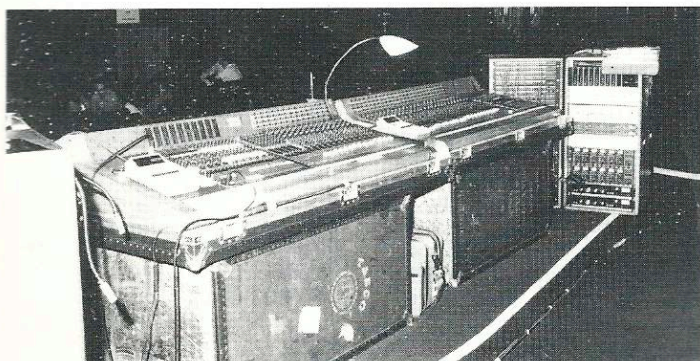
La console Midas/Tasco réalisée sur mesure.
