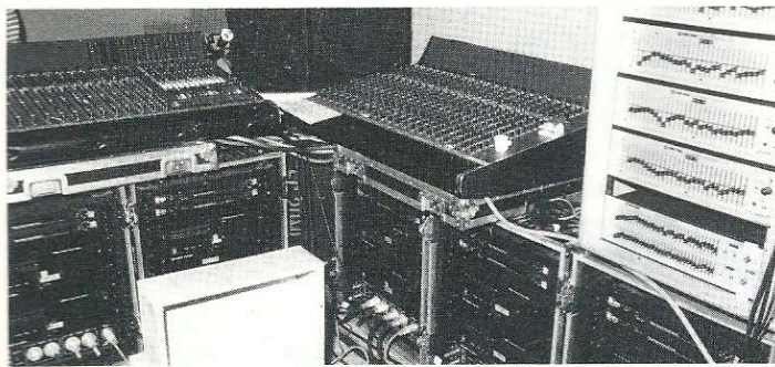
Sur scène, les retours. Sous les consoles, quelques amplis Crest Audio pour alimenter un tout nouveau système John Meyer encore top secret. Dans le haut de chaque rack d'amplis, les processeurs John Meyer.
